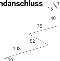
Wandanschluss
